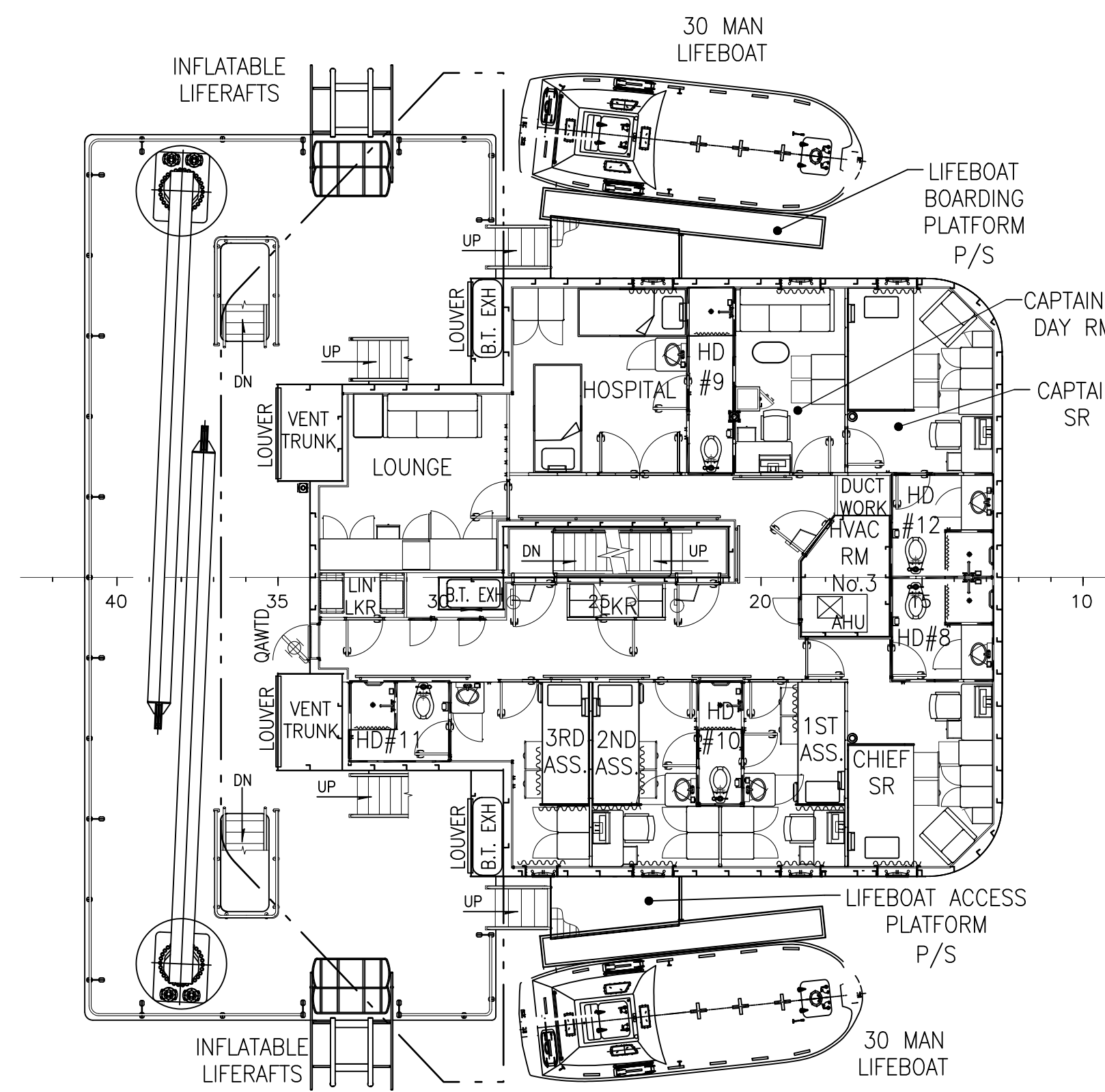
02 DECK SCALE: 1/8"=1'-0"
