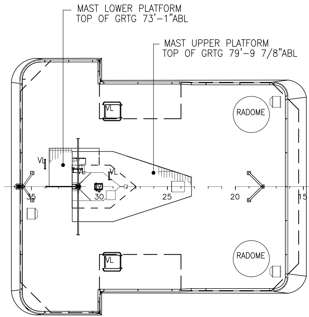
PILOT HOUSE TOP SCALE: 1/8"=1'-0"
