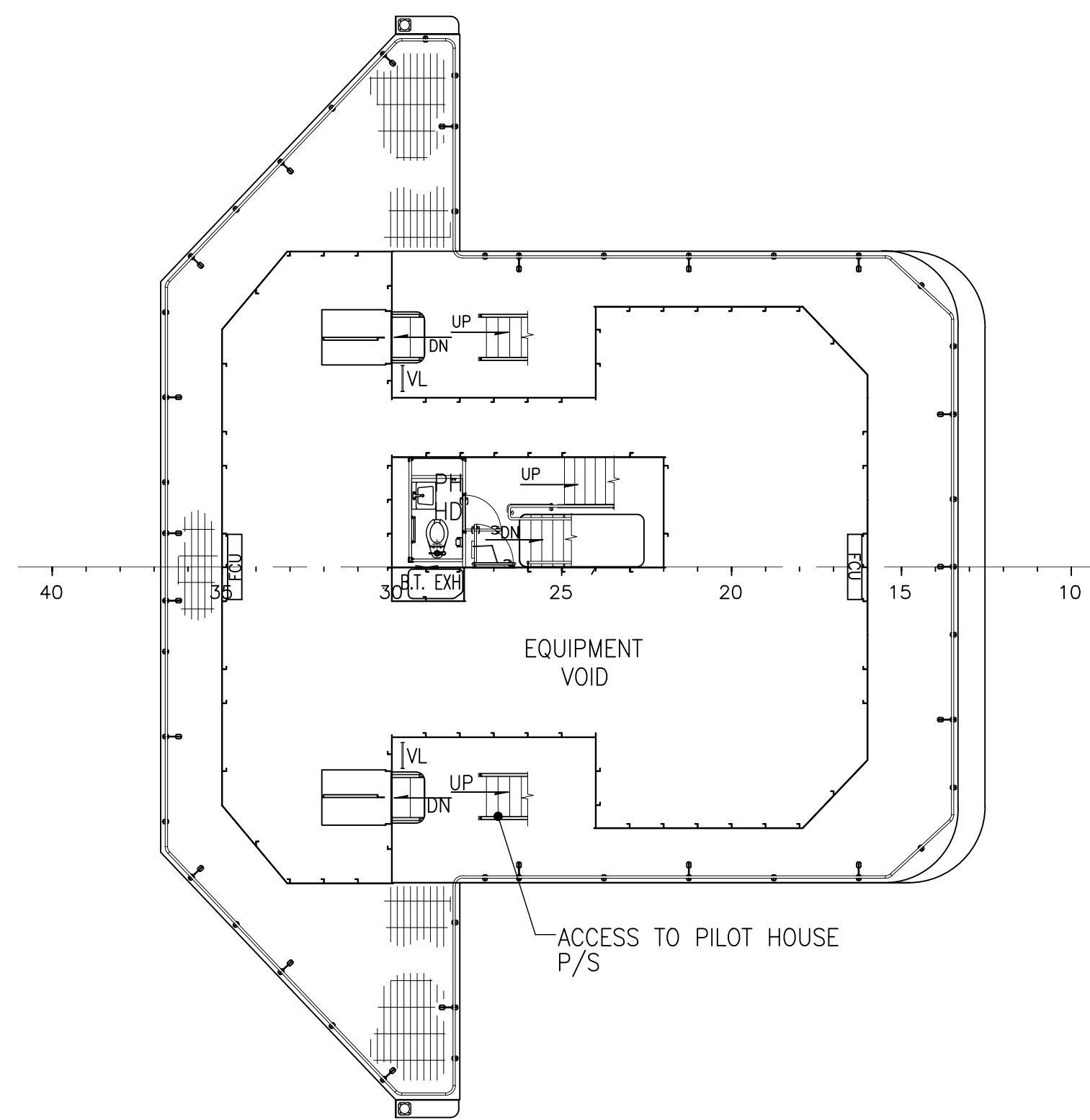
03 DECK SCALE: 1/8"=1'-0"
